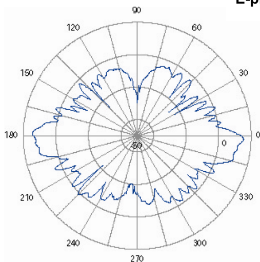
E-plane
