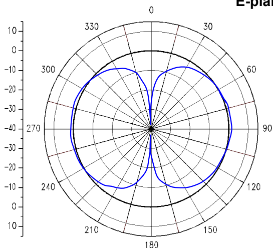
E-plane
