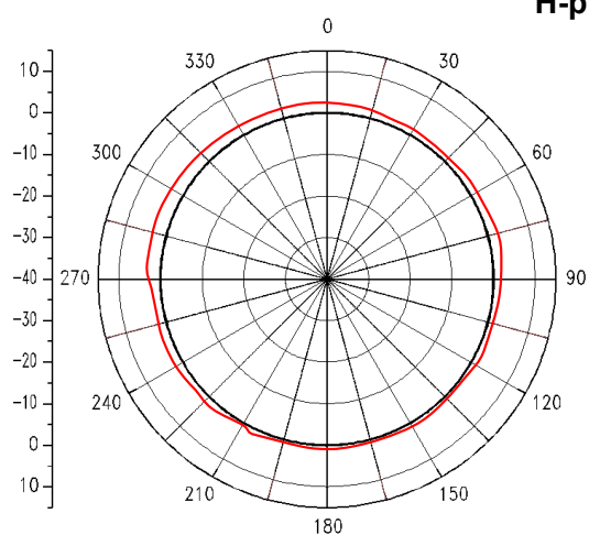
H-plane
