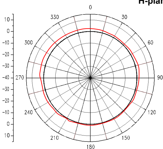
H-plane
